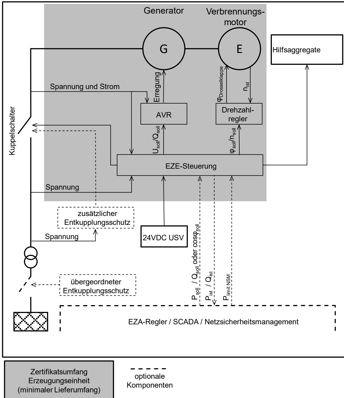
Abbildung 1: Schematisches Übersichtsbild der EZE SES HPC (Baureihe) (Quelle: Herstellererklärung 2025-03-07 ID165825 [D-3.3])
