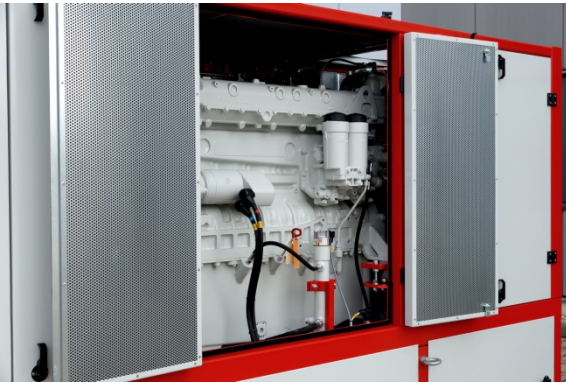
Hocheffizientes BHKW-Kompaktmodul SES-HPC 150 N Foto: SES Energiesysteme GmbH | Uwe Heinze
